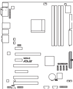
M2N-E IDE-Anschluss
