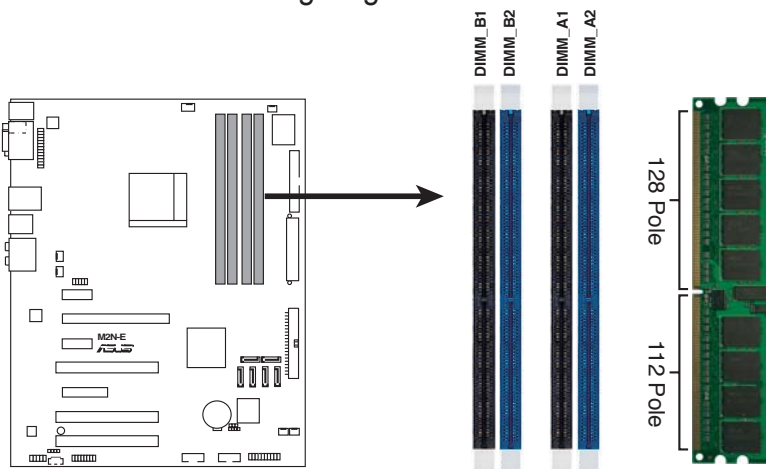
M2N-E 240-pol. DDR2 DIMM-Steckplätze
