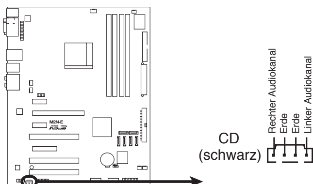
M2N-E Interner Audioanschluss
