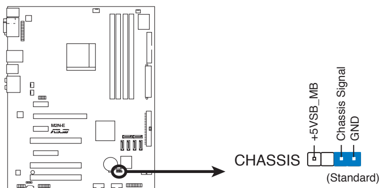
M2N-E Gehäuseeinbruchsanschluss
