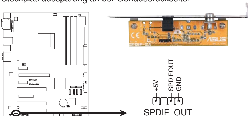
M2N-E Digitaler Audioanschluss
